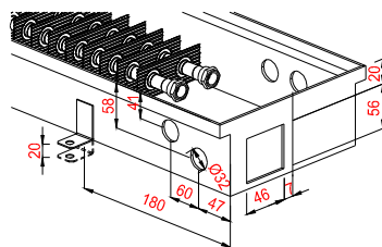
KORAFLEX FV 8/16
