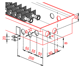
KORAFLEX FV 8/28 A=50, B=50 KORAFLEX FV 9/28 A=50, B=80
