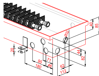
KORAFLEX FI 13/34
