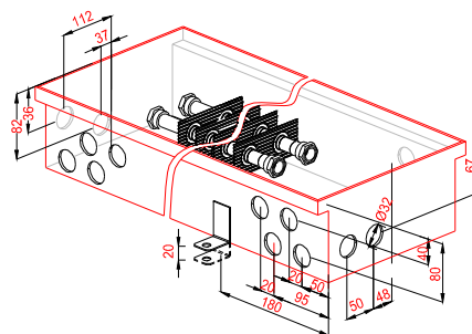
KORAFLEX FW 13/34
